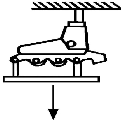
그림 6 신발의 부착강도시험
