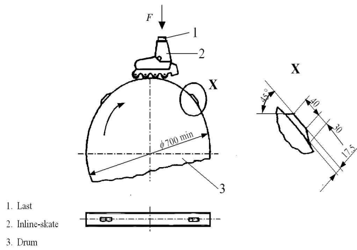
그림 5 주행시험
