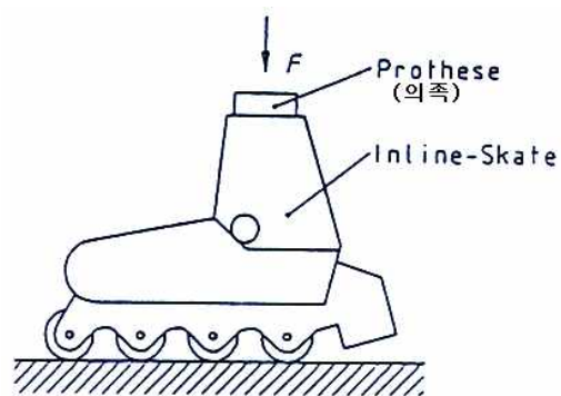
그림 7 압축하중시험
